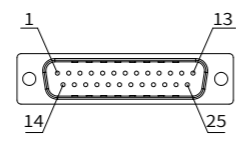
DB25公头(跳线)
