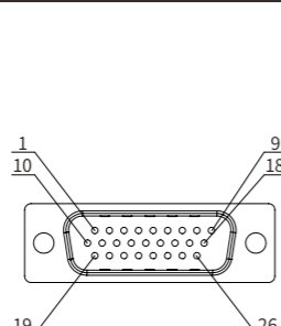
DB26公头
